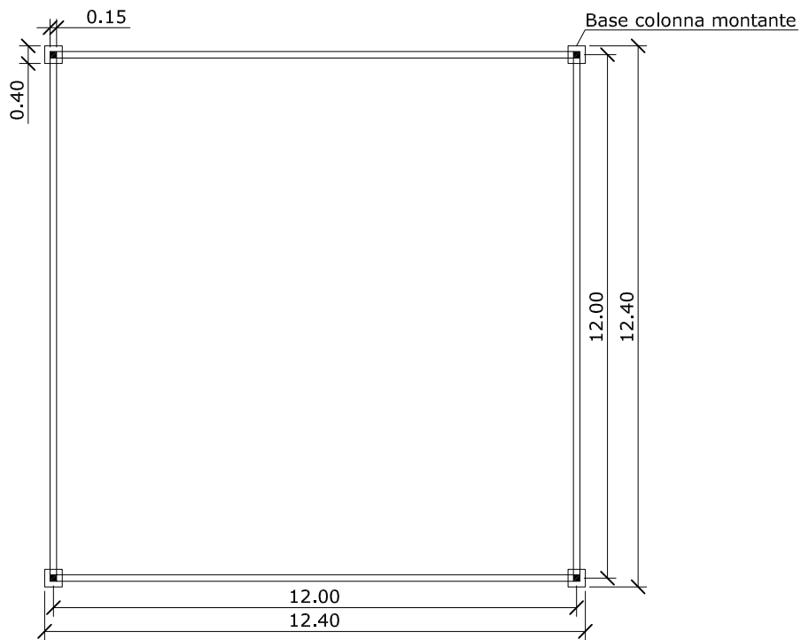
- PIANTA
