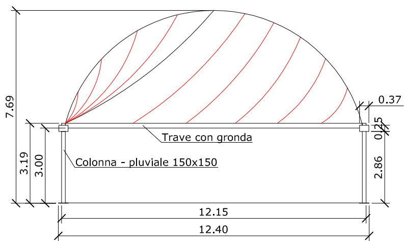
- PROSPETTO
